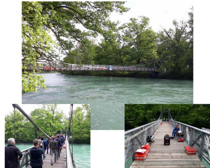
Schwingungsmessungen am Schönausteg, Bern
